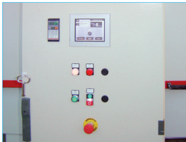
Quadro elettrico - Electrical board
